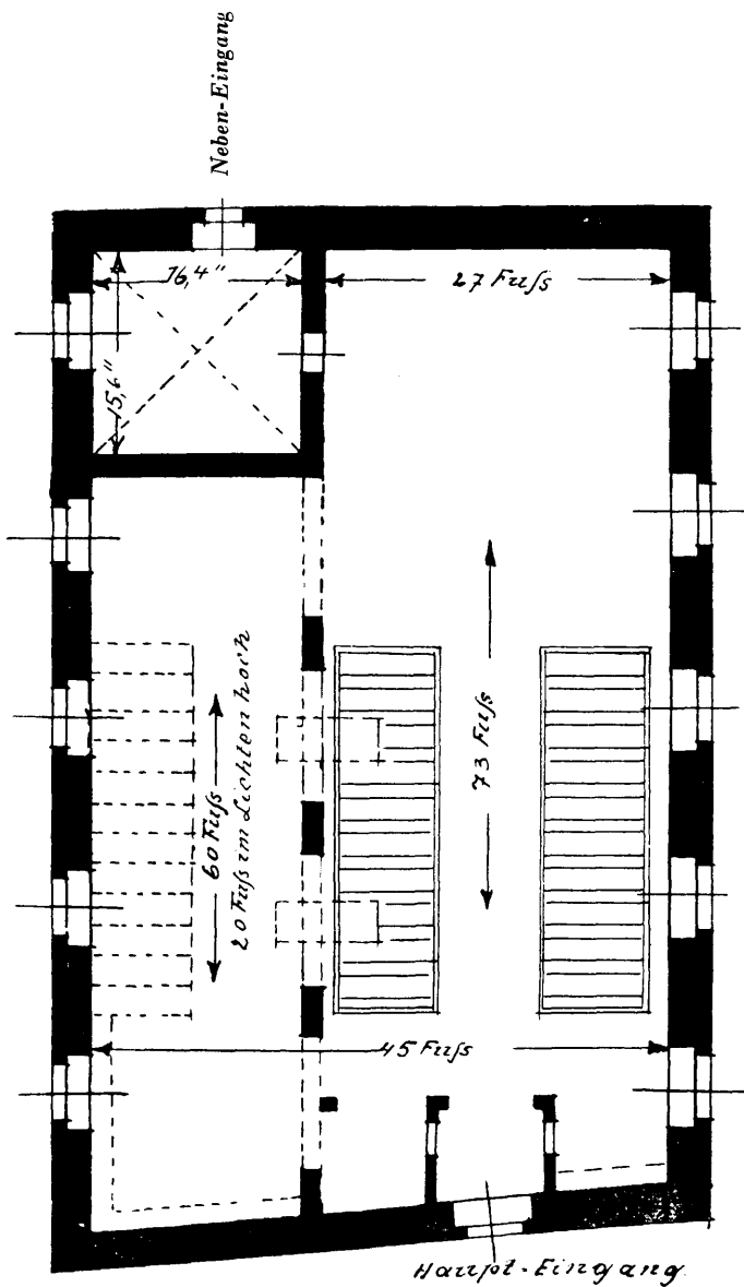
Grundriss der St. Anna-Kirche in Posen, 1816.
