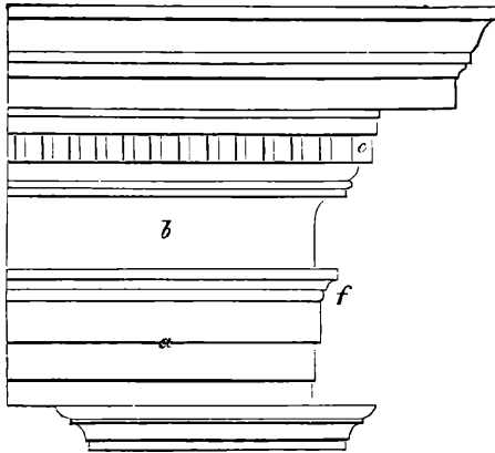
Fig. 39. Ionischer Oberbau.
