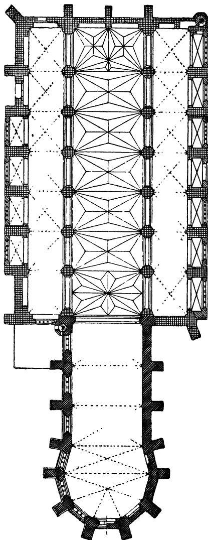
Fig. 2. Grundriß. 1 : 500. (Nach Suttö, Bausteinbauten, S. 12).
