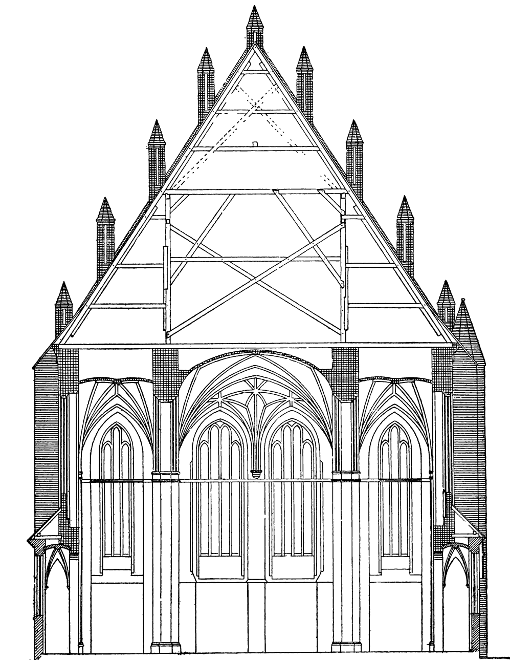
Fig. 3. Querschnitt des Langhauses mit dem Blick nach Westen. 1 : 225. (Nach Lutsch, Backsteinbauten, Tafel VII).
