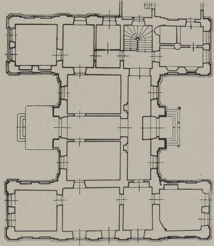
Schloß Groß-Holstein bei Königsberg Nach den Aufmaßzeichnungen des Provinzial-Denkmalamtes
