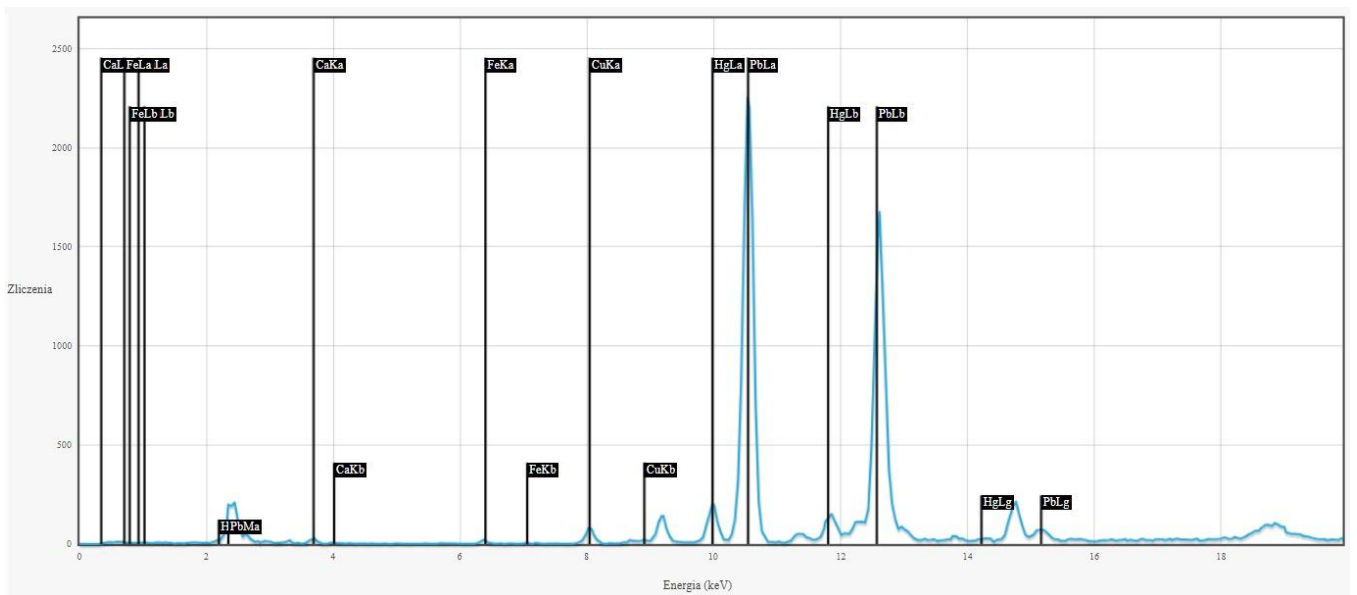
Rentgenowska analiza fluorescencyjna, pomiar w punkcie 4: Pb, Cl, Ca, Cu, Fe
