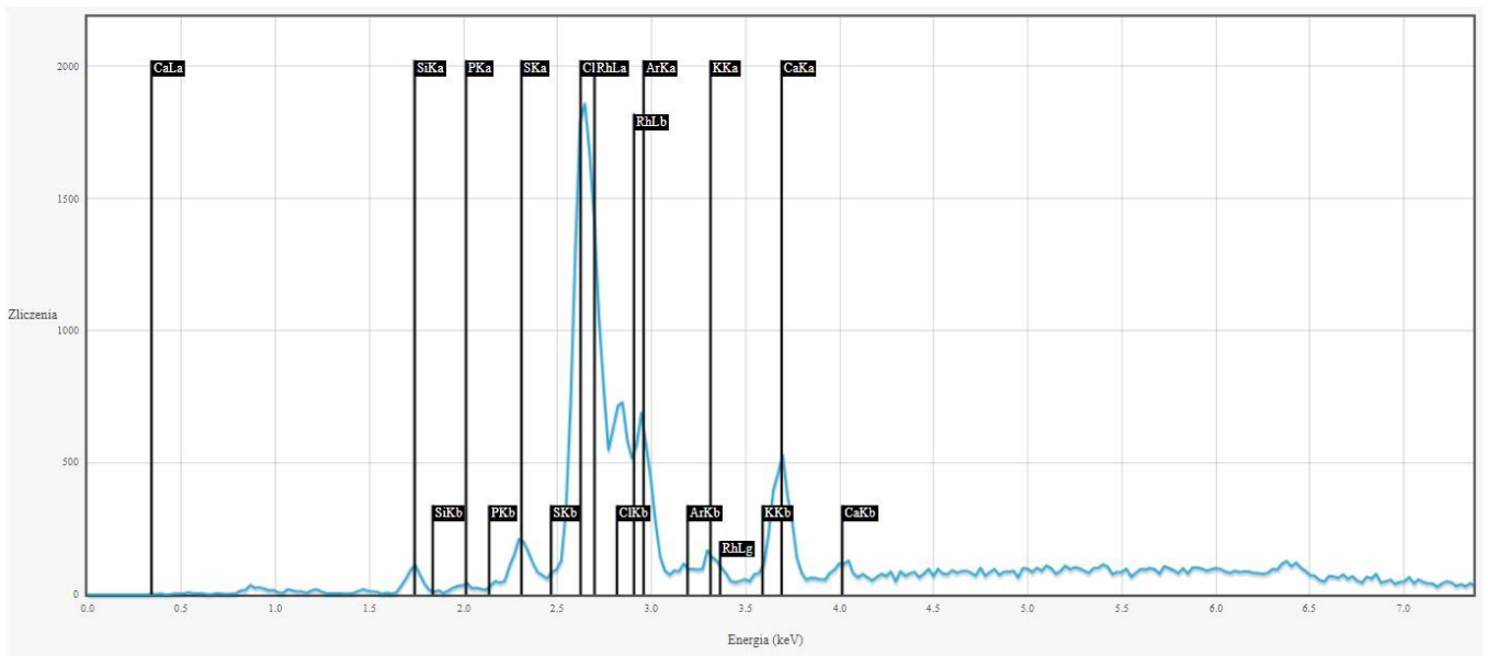
Rentgenowska analiza fluorescencyjna, pomiar w punkcie 3: Cl, Ca, K, Si
