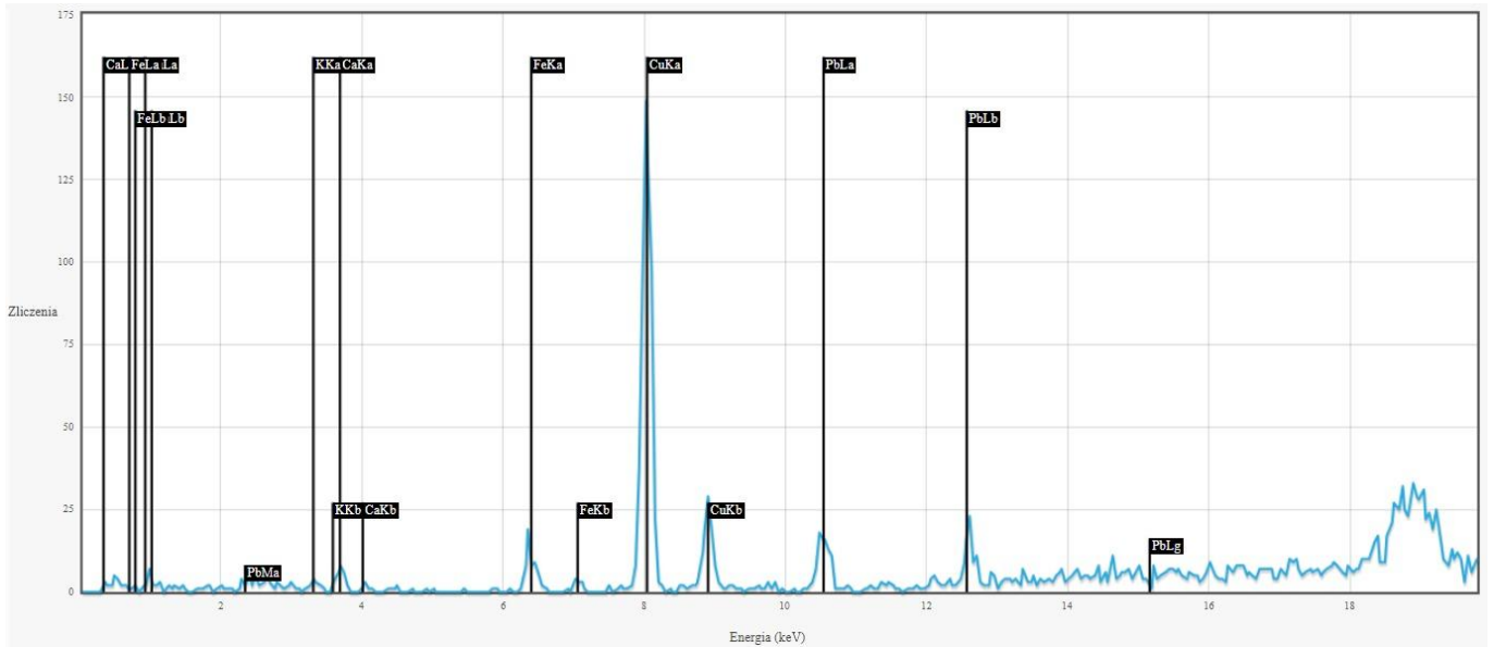
Rentgenowska analiza fluorescencyjna, pomiar w punkcie 10: Cu, Pb, Fe, Cl, Ca, K
