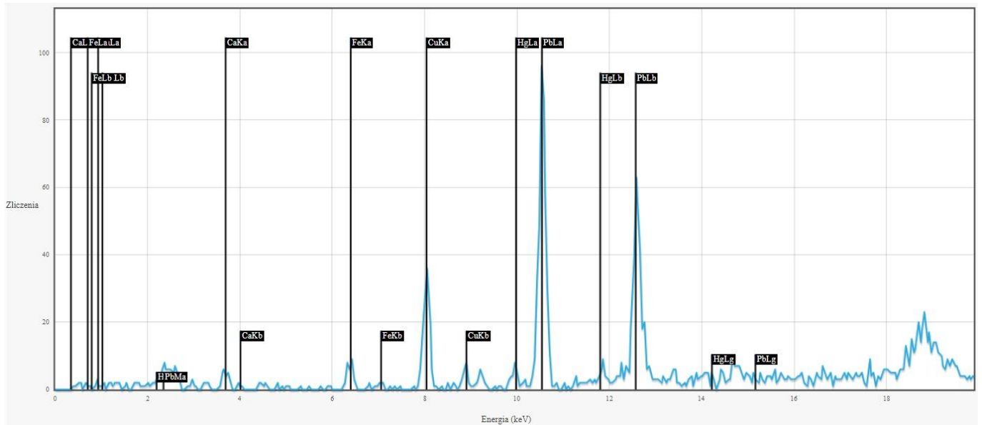
Rentgenowska analiza fluorescencyjna, pomiar w punkcie 2: Pb, Cu, Cl, Fe, Ca, Hg, S, K, Si, Al
