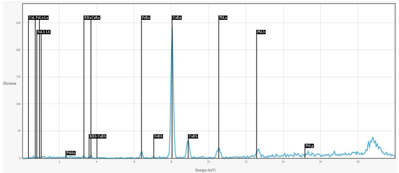
Rentgenowska analiza fluorescencyjna, pomiar w punkcie 8: Cu, Pb, Fe, Cl, S, Ca, Al, Si, S, P
