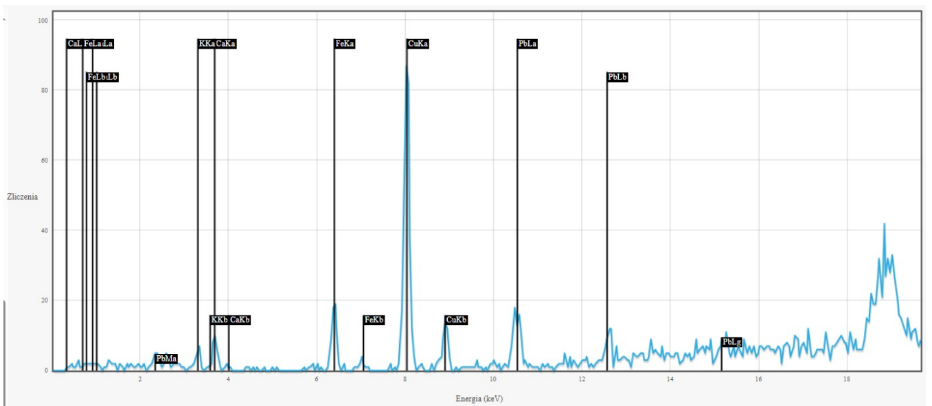
Rentgenowska analiza fluorescencyjna, pomiar w punkcie 11: Cu, Pb, Fe, Cl, Ca, S, K, Si, Al.
