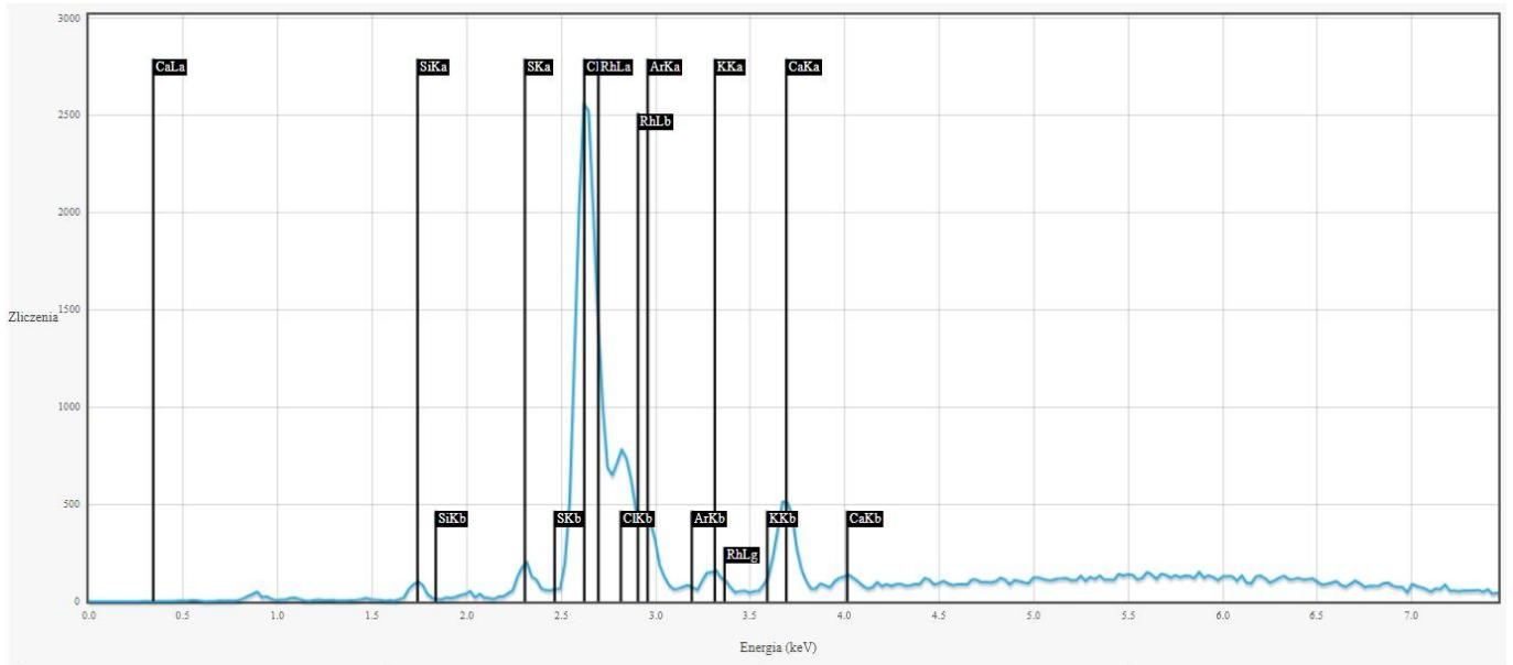
Rentgenowska analiza fluorescencyjna, pomiar w punkcie 12: Cl, Ca, K, S, Si
