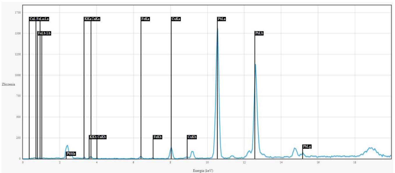
Rentgenowska analiza fluorescencyjna, pomiar w punkcie 5: Pb, Cu, Fe, Ca, K
