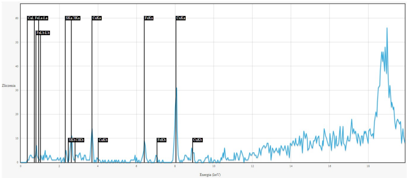
Rentgenowska analiza fluorescencyjna, pomiar w punkcie 13: Cu, Fe, Cl, Ca, S, Si, K, P
