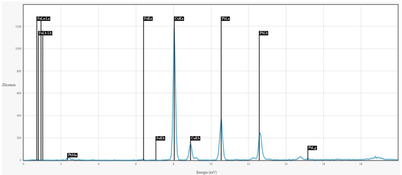
Rentgenowska analiza fluorescencyjna, pomiar w punkcie 7: Cu, Pb, Fe, Cl, S, K, Si
