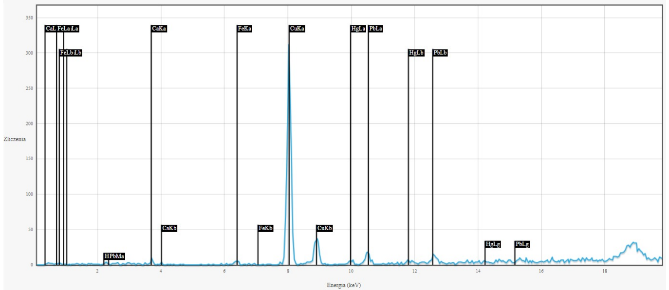
Rentgenowska analiza fluorescencyjna, pomiar w punkcie 9: Cu, Pb, Hg, Fe, Cl, S, Ca, Si, P
