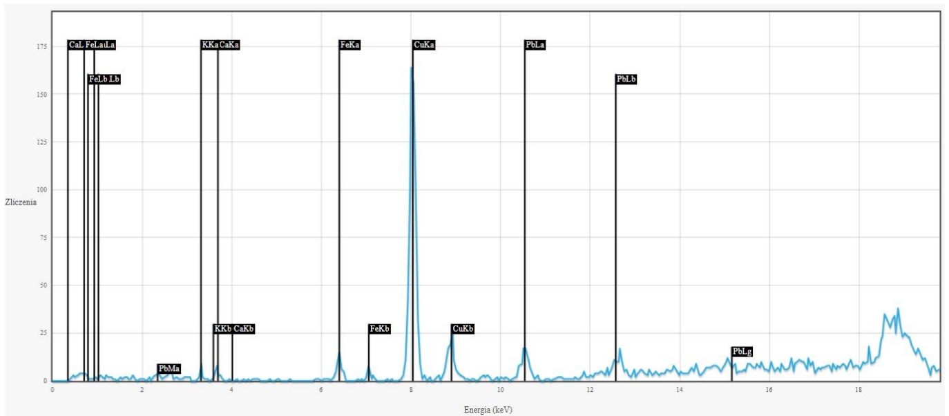
Rentgenowska analiza fluorescencyjna, pomiar w punkcie 6: Cu, Pb, Fe, Cl, S, Ca, Si, Al
