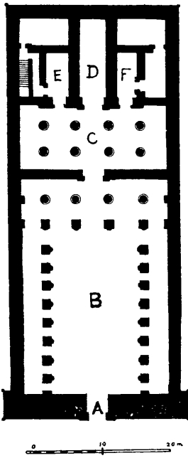
Tempel dem Amon Ré e in Karnak von Ramses III. errichtet, als Beispiel des gewöhnlichen Typus: A. Pylon. — B. Hof. — C. Hypostyl. — D. Kapelle des Amon. — E. Kapelle der Mut. — F. Kapelle des Chons. Die beiden letzteren mit Seitenräumen, deren einer die Treppe zum Dach enthält.
