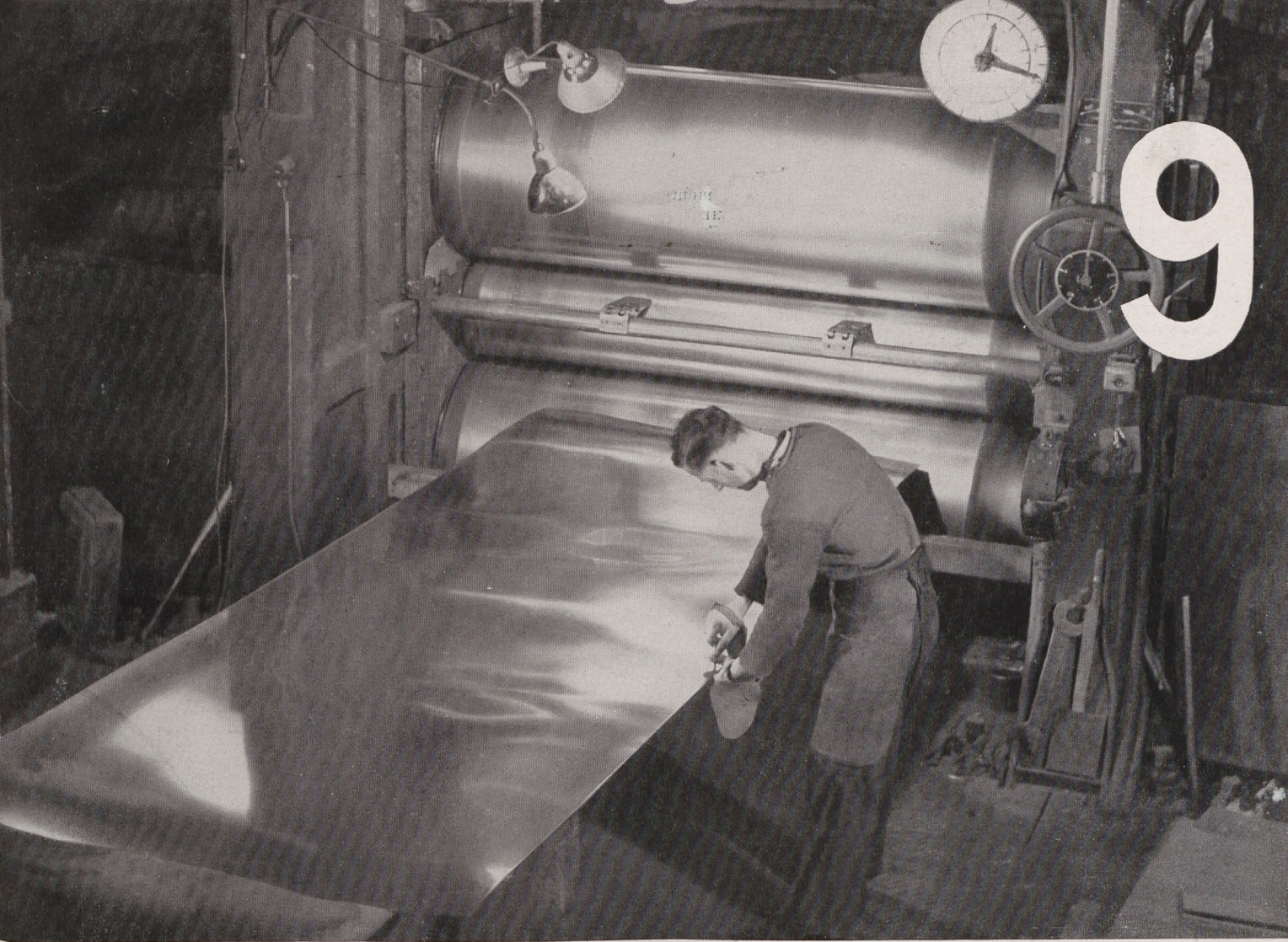
Stätten deutscher Arbeit: Kaltwalzen von Blechen aus Leichtmetall Duralumin auf einem Triogerüst im Werk Berlin-Borsigwalde der Dürener Metallwerke A. G.
