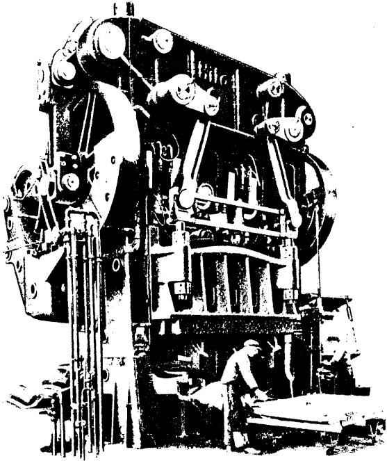
Schwere Kniehebel-Breitziehpresse für Karosserieletzte im Betrieb Maschinenfabr. HILTMANN & LORENZ AG. Aue i. Sa.
