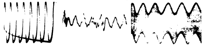
Links: Schwingungen von 240000 Hz mit einem Gleichlaufzang von 1:8 Mitte: Klangkurve eines „a“ - Lautes Rechts: Additive Modulation zwischen 50 Hz und 10000 Hz
