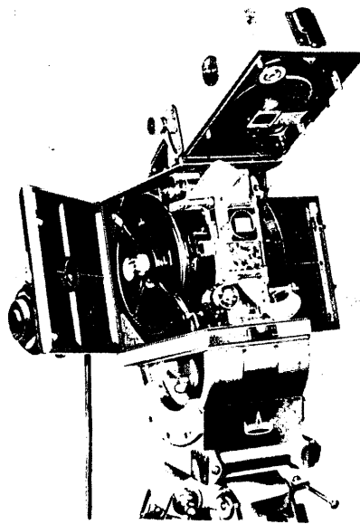
Abb. 11 Askania-Filmkamera für Normalfilm-Aufnahmen; die geöffneten Seitentüren und das hochgeklappte Vorderteil mit dem Objektiv lassen die Anordnung der Filmrollen (Kassetten) sowie das sogenannte Bildfenster und den Filmlauf erkennen
