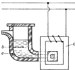
Abb. 5 Niederfrequenz-Induktionsöfen nach Kjellin
