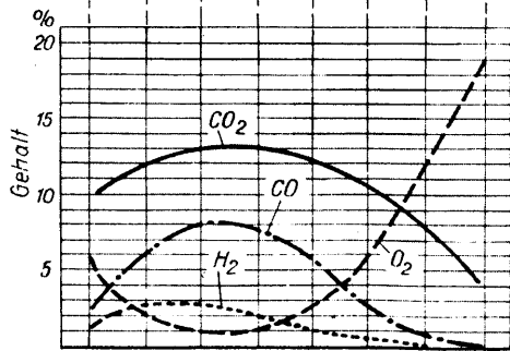
Abb. 1 Zusammensetzung der Feuegase über dem Brennstoffbett eines Zonenwanderrosts mit Unterwind
