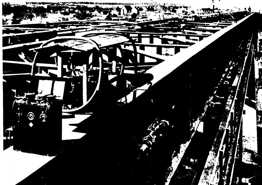
Abb. 21b Brückenuntersuchung mit Hilfe von Röntgenstrahlen
