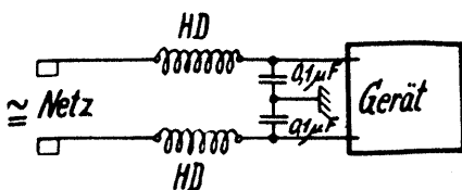
Abb. 12 Hochfrequenz-Sperrgitter mit eisenlosen Hochfrequenzdrosseln ( L = 0,8 \text{ mH} )
