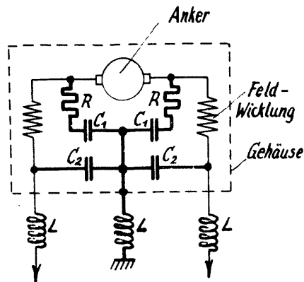
Abb. 14 Entstörung eines Hauptstrommotors. R, C 1 : Funkenlöschung, L, C 2 : Hochfrequenz-sperren gegen Netz und Erde
