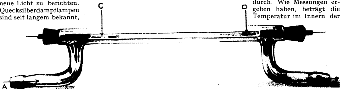
Abb. 3 Eine ältere Type der Philips-Hochdruck-Quecksilberdampf Lampen mit Wasserkühlung. Länge 15 cm, Lichtmenge 55000 Kerzen. A) Wasserzuführung, B) Wasserableitung, C) und D) Elektroden
