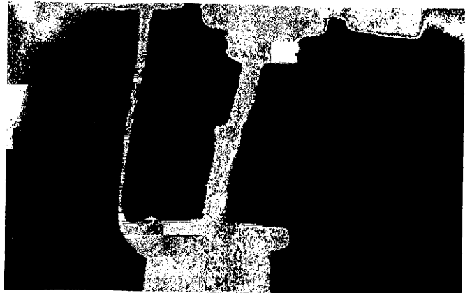
Abb. 33 Aufnahme eines Kabelendverschlusses. In der Vergußmasse hat sich ein kugelförmiger Hohlraum gebildet
