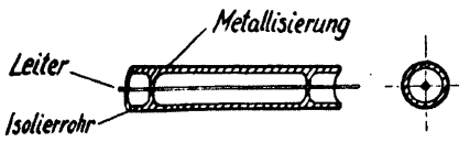
Abb. 10 Schnitte durch ein abgeschirmtes Antennenkabel
