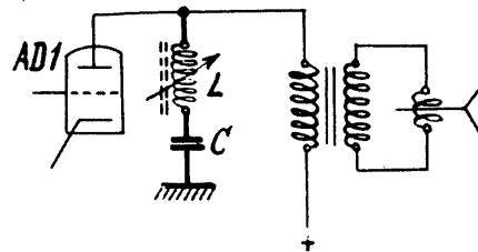
Abb. 13 Endstufe mit der Triode AD 1, einer 9-kHz-Sperre ( L = 0,1 \text{ H} , C = 3000 \text{ pF} ), dem Lautsprecher-Übertrager und der Schwing-spule eines dynamischen Lautsprechers
