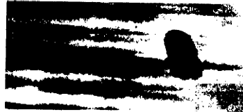
Abb. 30 Aststelle in einer Sperrholzplatte geröntgt. Bei Dicken über 2,5 mm ist eine Durchstrahlung mit starken Glühlampen nicht mehr möglich
