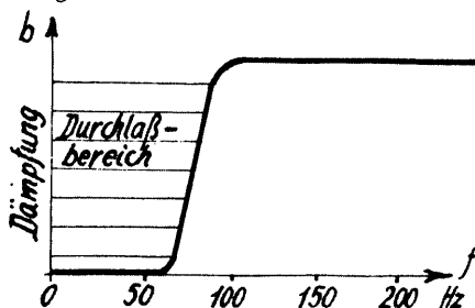
Abb. 8 Dämpfungskurve eines Niederfrequenz-Siebgliebes mit einer unteren Grenzfrequenz f_u = 60 \text{ Hz}
