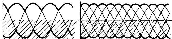
Abb. 6 Stromverlauf bei 3-Phasen-Gleichrichtung. Starke Welligkeit durch 3. Oberton
