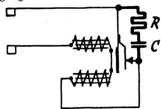
Abb. 15 Entstörung einer elektrischen Klingel durch Funkenlöschung (R, C)
