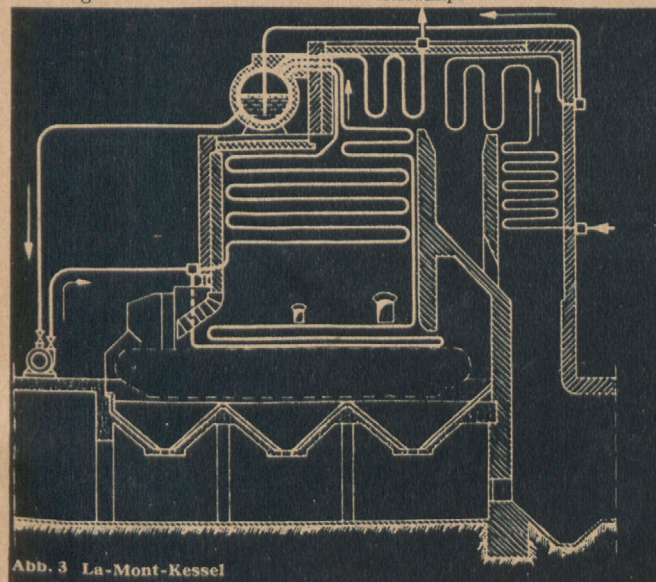
Abb. 3 La-Mont-Kessel
