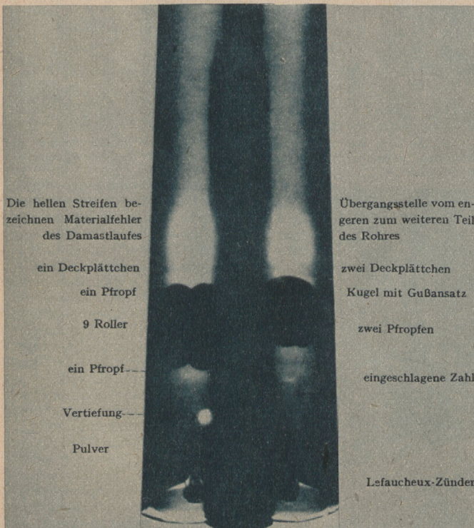
Abb. 2 Mit X-Strahlen durchleuchteter Gewehrlauf (Abb. 1); die erste Durchleuchtung eines metallischen Gegenstandes, von Röntgen selbst vorgenommen
