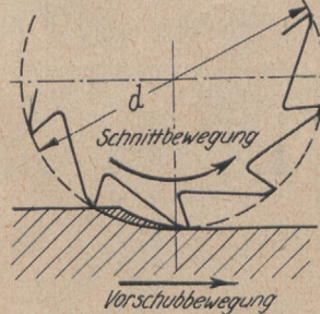
Gleichlauffräsen
