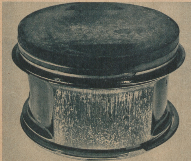
Abb. 2a Kolben hat infolge Überhitzung gefressen
