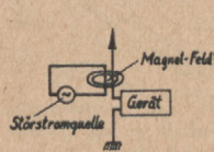
Abb. 3 Magnetische Störbeeinflussung an der Antenne
