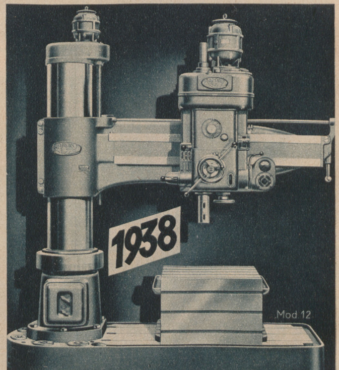
Abb. 9 Neuzeitliche Radialbohrmaschine mit 19 Bohrspindeldrehzahlen und 18 Vorschüben, die je mit nur einem Hebel geschaltet werden
