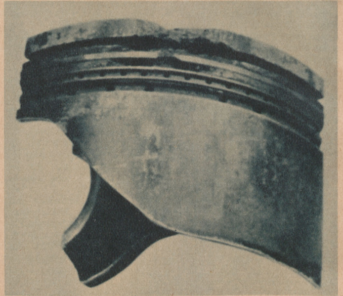
Abb. 2b Ausgebrannter Kolben infolge Überhitzung durch klopfenden Motorbetrieb
