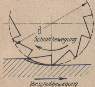
Gegenlauffräsen Abb. 3
