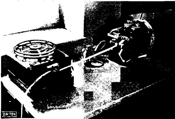
Bild 8. Registriergerät (Drehpulschnellschreiber) mit zwei Schreibfedern.
