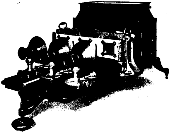
Bild 1. Projektionsapparat für Dreifarbenphotographie von C. P. Goerz nach Professor Dr. A. Miethe
