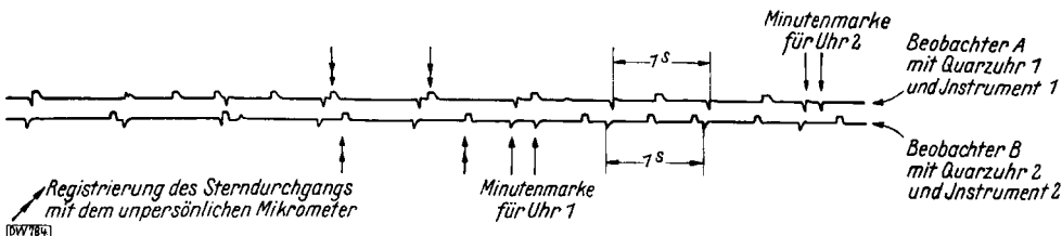
Bild 9. Registrierstreifen eines Drehspulsnellschreibers
