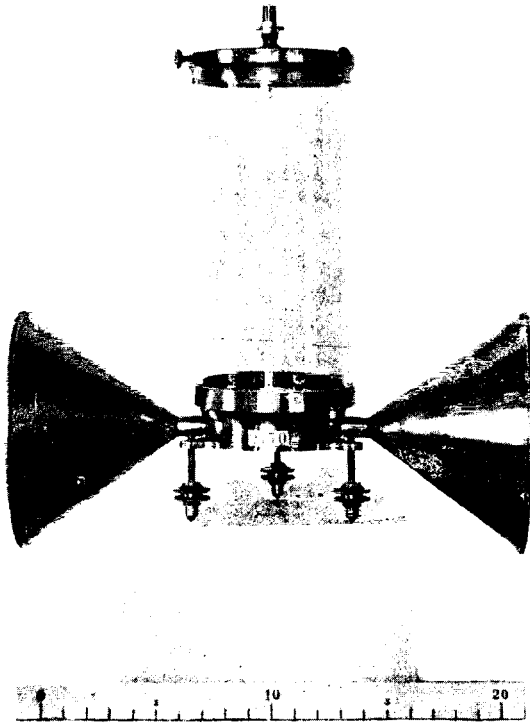
Bild 5. Ohms Melonische Säule mit Galvanometer
