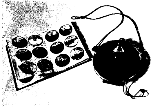
Bild 3. Knopflochkamera von C. P. Stirn, 1886
