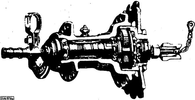
Bild 10. Torpedo-Freilaufnabe mit zwei Geschwindigkeiten
