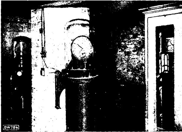
Bild 5. Luftdichte Pendeluhren von Cl. Riefler im Uhrenkeller des Geodätischen Institutes in Potsdam
