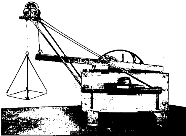
Bild 2. Kalorischer Kraftmesser von J. R. Mayer, 1868 Länge des Bremsbalkens 220 cm
