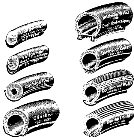
Bild 6. Entwicklung der Gummibereifung
