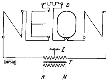
Abb. 10. Hochspannungs-Leuchtröhrenschialtung
