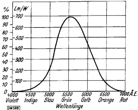
Abb. 2. Relative Werte der Augenempfindlichkeit und photometrisches Strahlungsäquivalent in Abhängigkeit von der Wellenlänge
