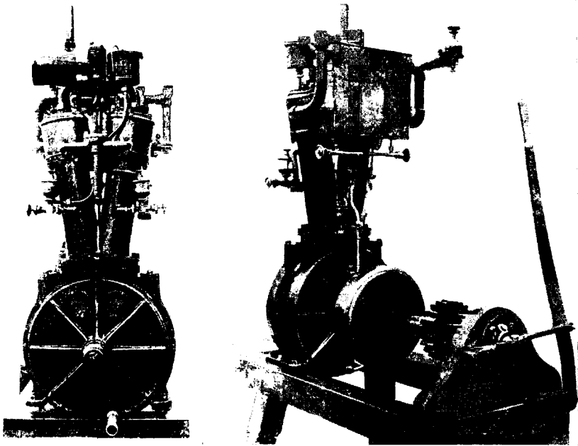
Abb. 8. Daimlers Motor mit V-förmig angeordneten Zylindern, 1889
