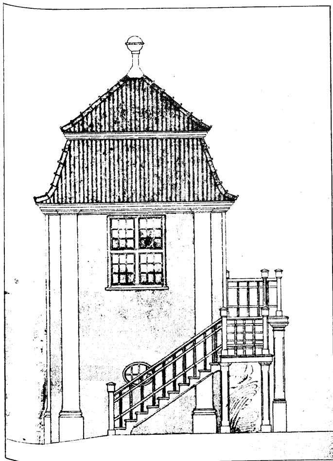
Abb. 8. Gartenhaus Konradshammer, nach einer Aufnahme des Kgl. Hochbauamts Danzig II. Maßstab 1:100.
