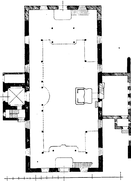
Abb. 4a. Evang. Kirche Groß Nebrau, jetziger Grundriß, nach einer Zeichnung des Kgl. Hochbauamts Marienwerder. M. 1:400.
