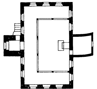
Abb. 4b. Grundriß der Kirche in Dakau. M. 1:400.
