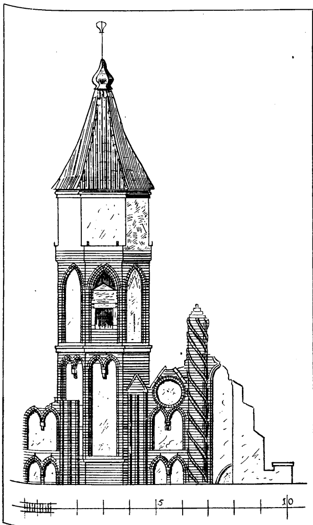
Abb. 11. Südgiebel des Rathhauses zu Strasburg. Maßstab 1 : 150.
