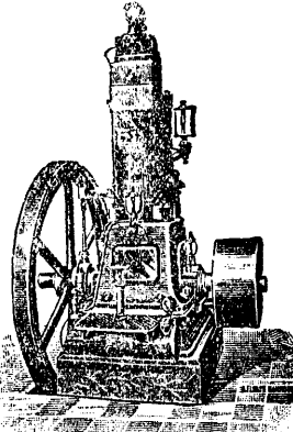
Stehende Anordnung. Modell H.
