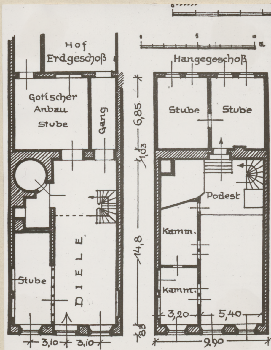
2. Kamieniczka nr 3. Rzut parteru i II kondygnacji rys. Rendschmidt, o.c., 54. 58-59
